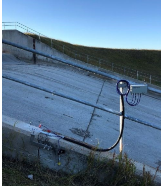
Suivi des fissures sur le déversoir
