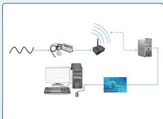
• Principe de fonctionnement de la station
